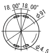
取付穴位置
