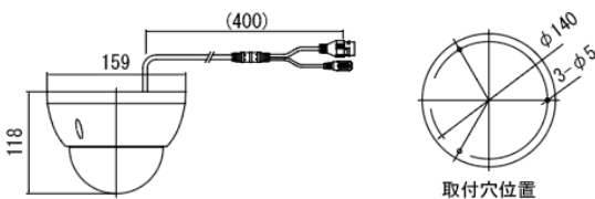
取付穴位置
