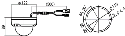
取付穴位置
